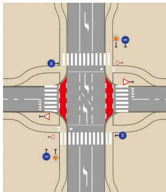
Fietsgeleiding op een kruispunt zonder verkeerslichten (met haaiantanden)
