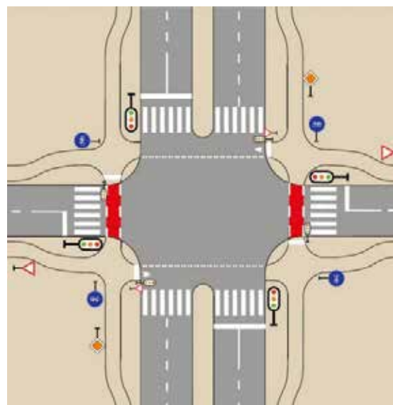
Fietsgeleiding op een kruispunt met verkeerslichten (met stopstrepen)
