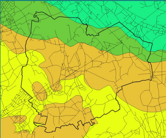
Geologische kaart van Kampenhout. De gele band markeert de insnijding van de oude rivier doorheen de Lediaan-formatie (oranje) tot in het Brusseliaan (geel).
